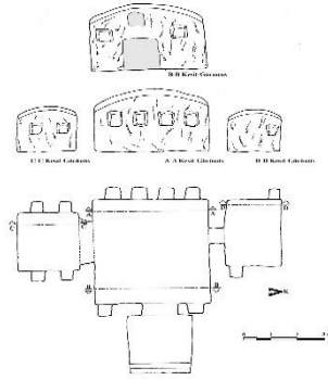
Çizim 3. Yoğunhasan Kaya Mezarı Planı
