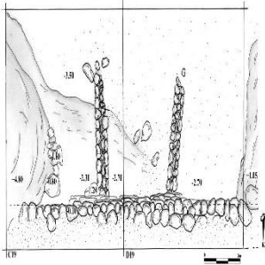
Çizim 8. Pasinler Kalesi Urartu Sur Duvarı
