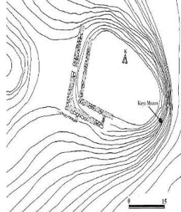
Çizim 1. Yoğunhasan Kalesi Planı
