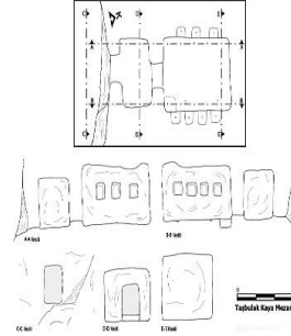
Çizim 17. Taşbulak Kaya Mezarı
