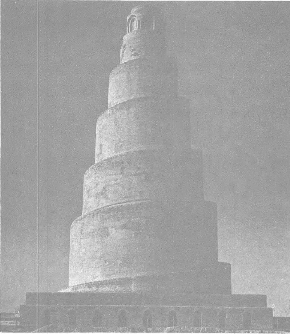
Samarra'daki Büyük Camiin helezonî minaresi. Abbasiler tarafından IX. yüzyılda kurulmuş olan Samarra kentindeki bu cami, çok değişik bir mimari yapıya sahiptir.
