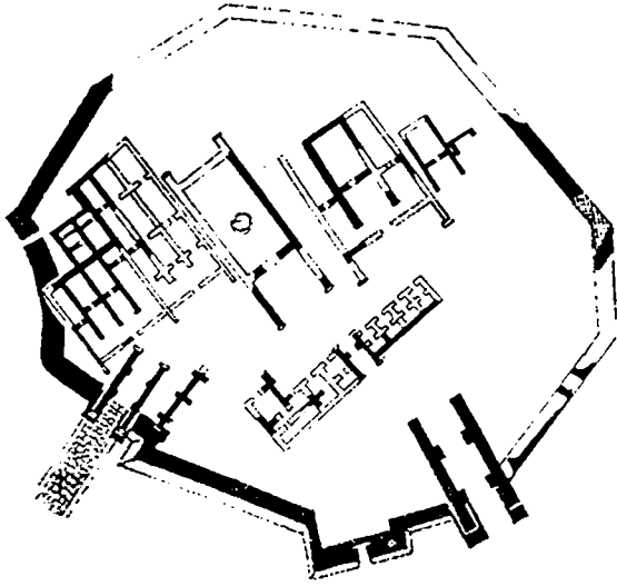
II. Troia kalesi planı
