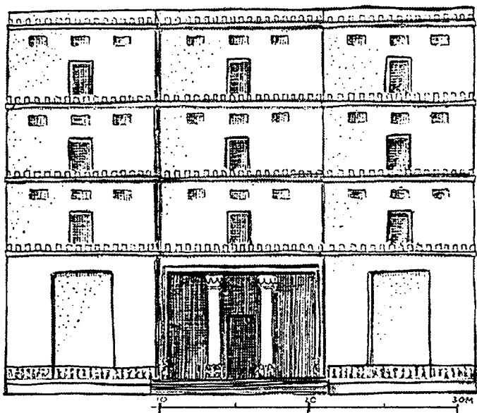
Bir Bū-Hilani'nin cepheden görünüşü
