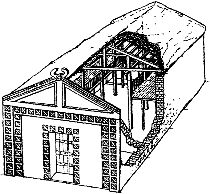
Gordion Megaron 3'ün rekonstrüksiyonu
