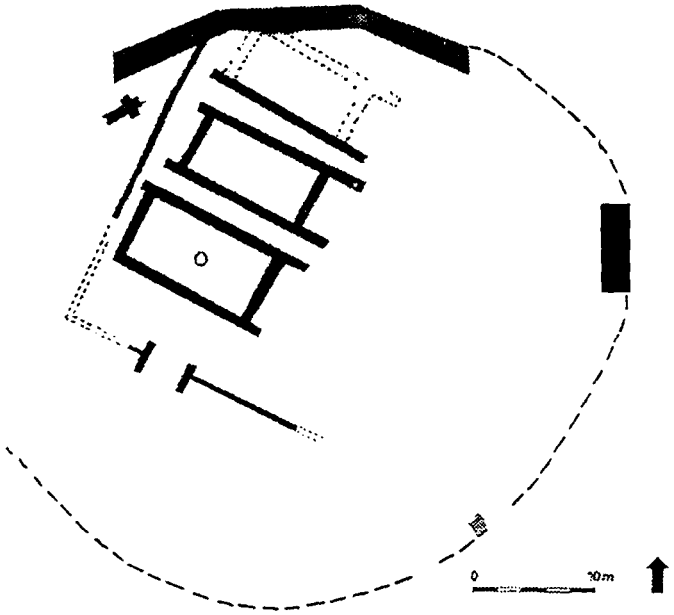
Kanlıgeçit Kalesi planı
