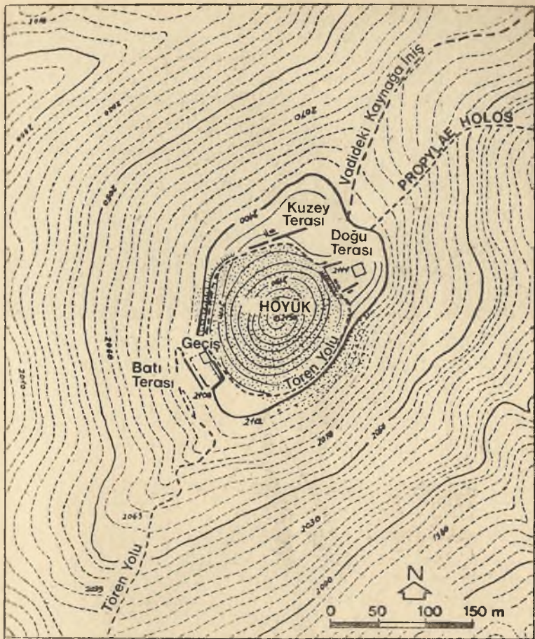
Şekil — 2 : Nemrud Dağı Açıkhava Mabeti'nin plânı. (Bn. Theresa Goell'e göre.)
