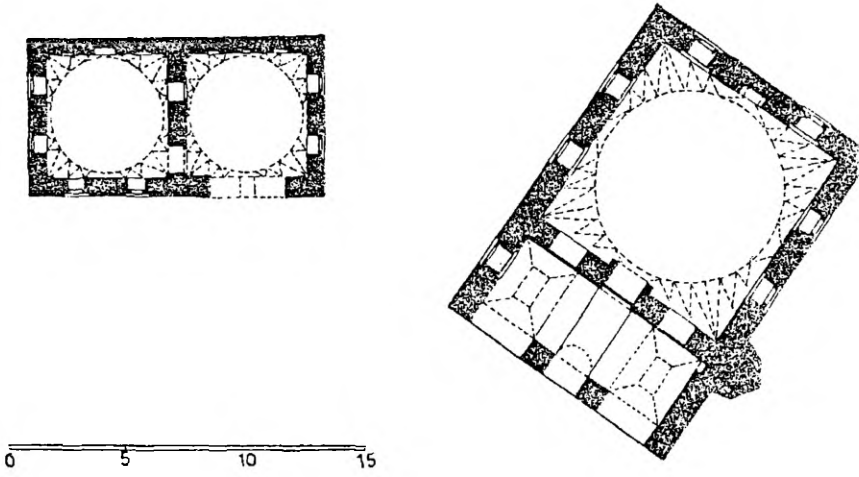
No: 38-39-Bursa'da (Atpazarı semtinde) Sitti Nefise Hatun Mescidi ile Mektebi'nin temel plânları.
