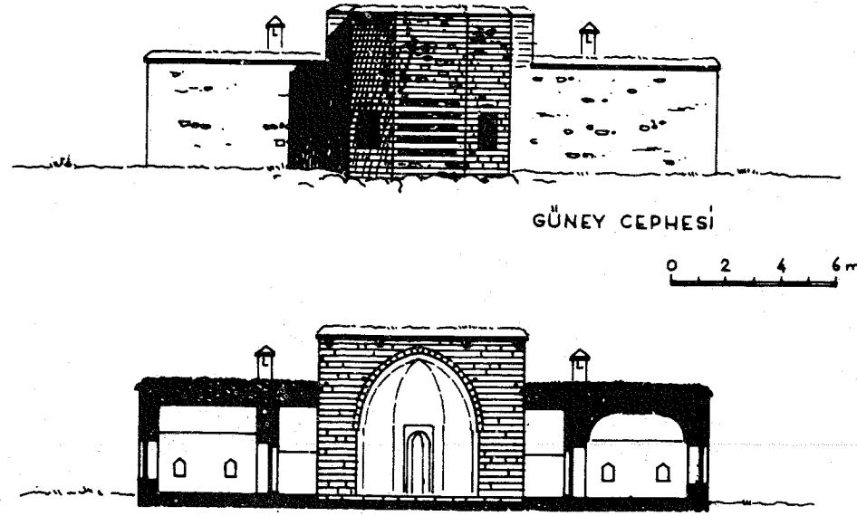
Çizim 16 – Medreseden enine kesit (O. C. Tunçer)
