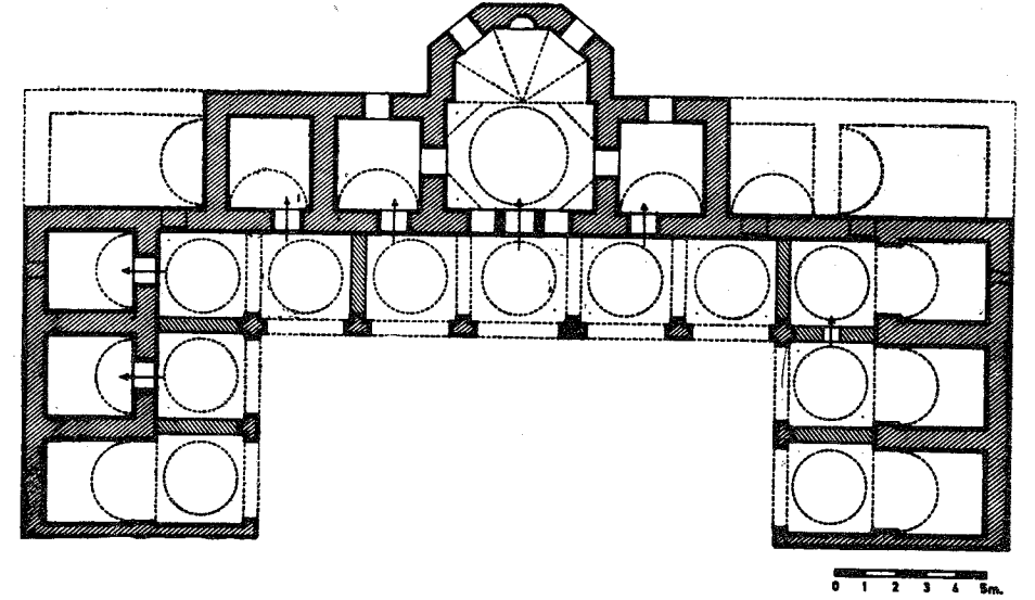
Çizim 19— Çeteci Abdullah Paşa Medresesi Planı (R.H. Ünal'dan)
