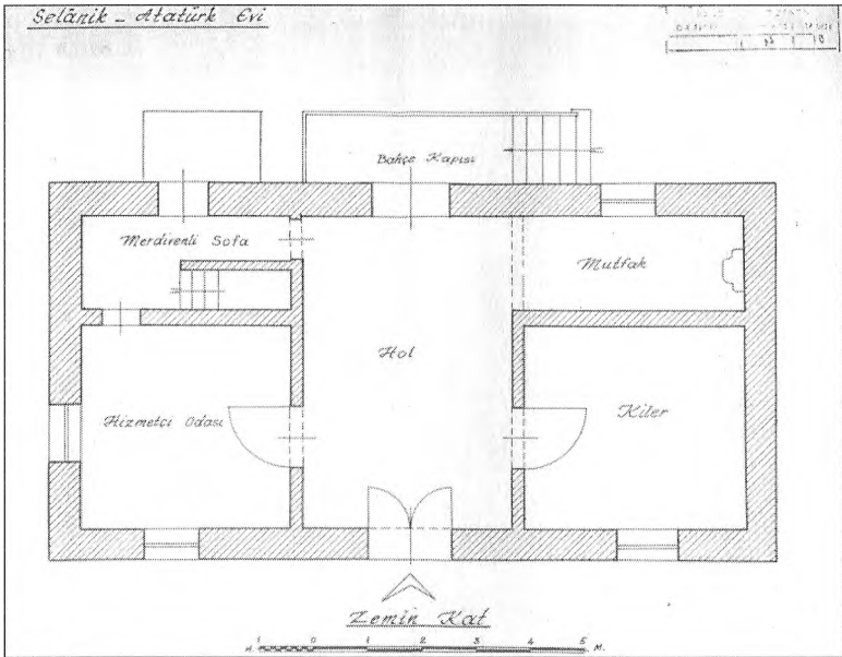
Selânik Atatürk Evi'nin Planları
