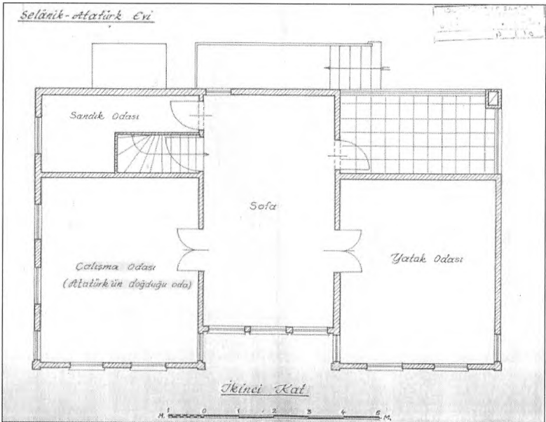
Selanik Atatürk Evi'nin Planları
