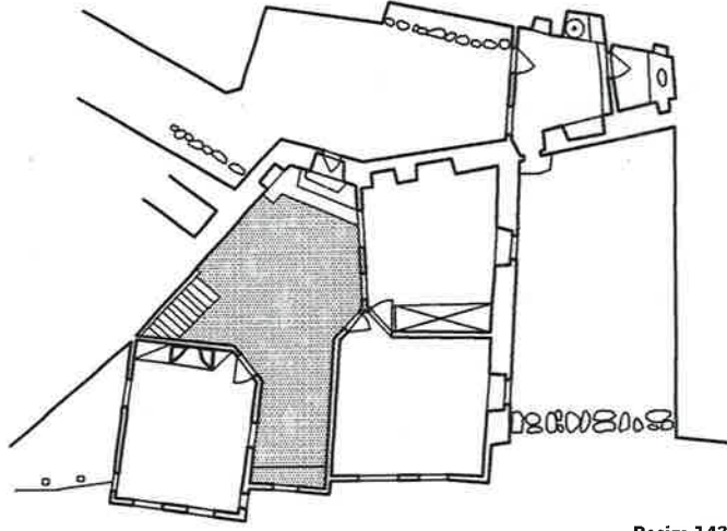
Resim 143. Midilli. Molyvos'ta Bagladania Evi üst kat planı ve giriş cephesi.
