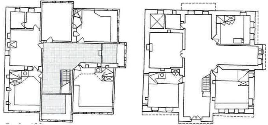
Resim 190. İpek'te Kasapoli Evi'nin kat planları.
