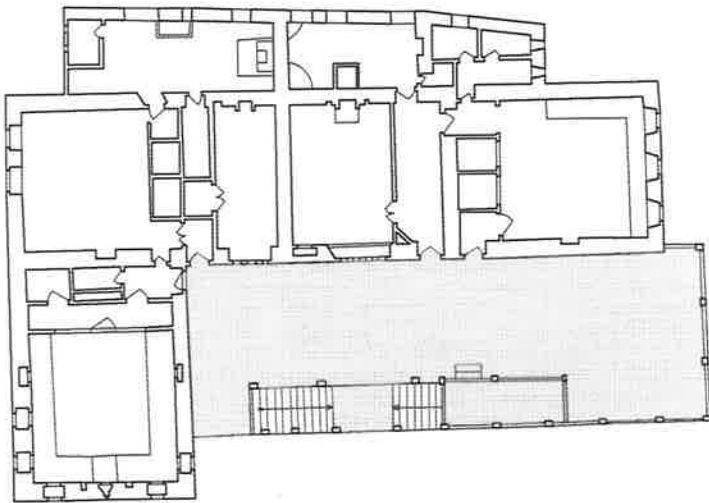
Resim 263. İşkodra'dan Ymer Ramadan Evi. Kat planları ve görünüşler.
