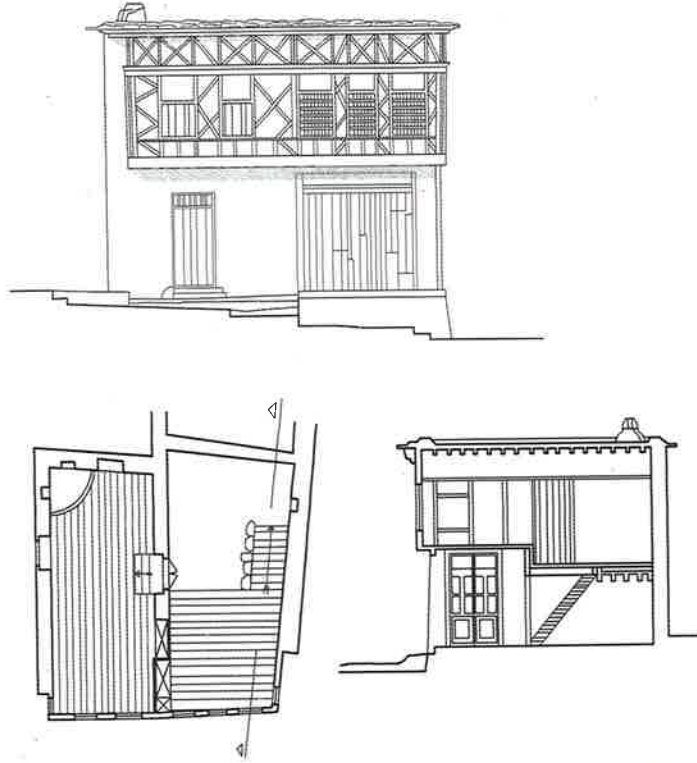
Resim 150. Sisam, Nichori'de Sariyannis Evi kat planı, kesit ve giriş cephesi.
