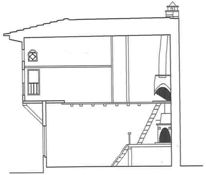
Resim 149. Sisam, Pano Vathy'de K. Tsopanarias Evi kat planları ve kesit.
