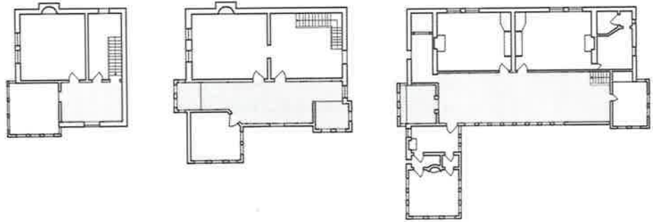
Resim 23. Rodop evlerinde köşklü üst kat planları.
