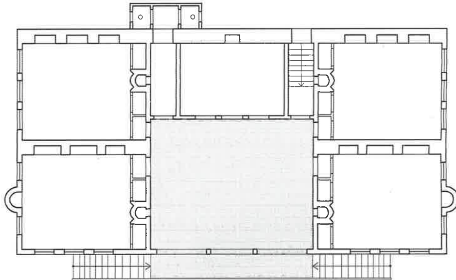
Resim 179. Kalkandelen'den bir bey evi. Üst kat planı ve avlu cephesi.
