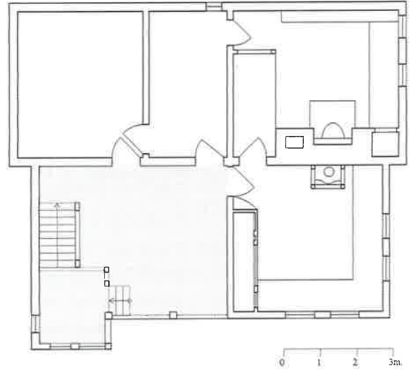
Resim 17. Koprivštitsa'dan dış sofalı/köşklü ev planı.
