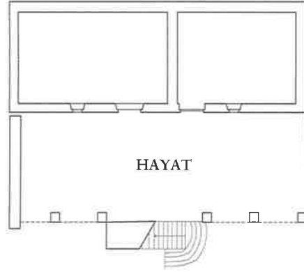
Resim 259. İşkodra'dan çardaklı bir ev. Kat planları ve görünüşü.
