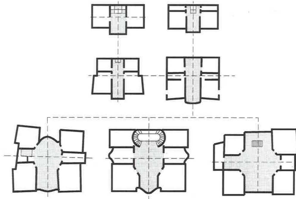
Resim 59. Filibe tipi kapalı simetrik evlerin gelişim şeması.
