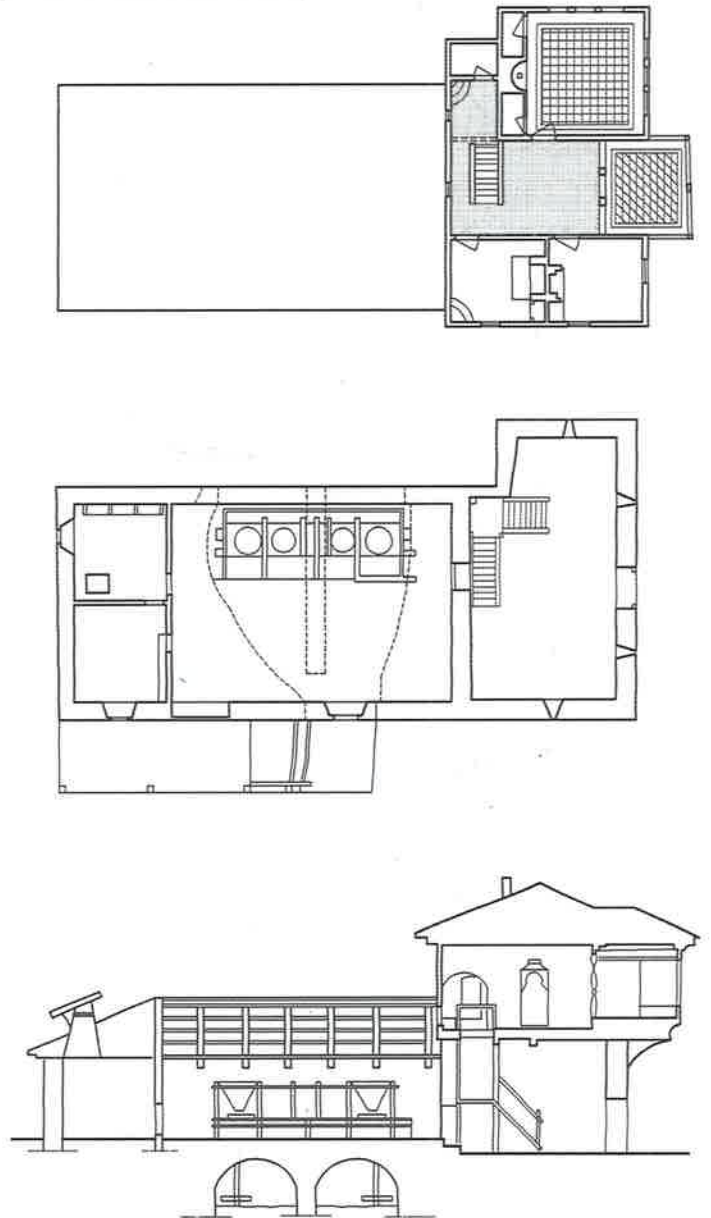
Resim 215. Pirot'tan bir su değirmeni ve konut kısımının kat planları ve kesiti.
