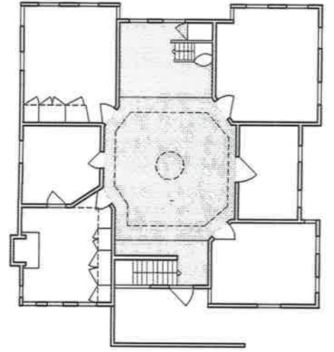
Resim 46. Nessebar'da Muskoyanın ve Küçükün Evi kat planları.
