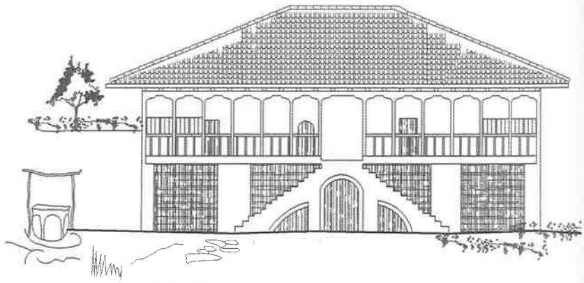
Resim 260. İşkodra'dan çardaklı bir ev. Kat planları ve görünüşü.
