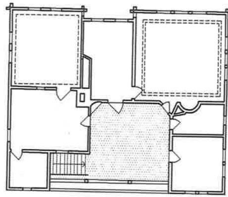
Resim 37. Triavna'da Raikov Evi üst kat planı.
