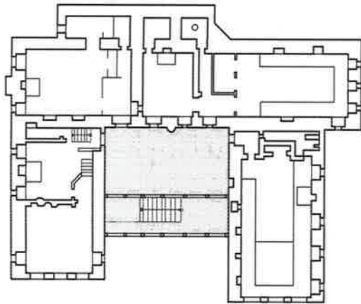
Resim 283. Ergeri'den kule tipi ev. Kat planları ve görünüş.
