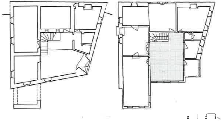
Resim 151. Sisam, Chora'da konak. Kat planları.
