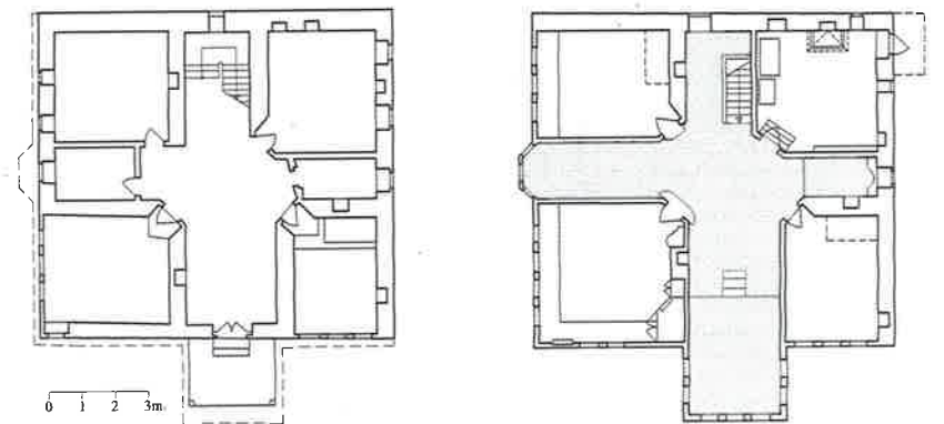
Resim 192. İpek'te Protić Evi'nin kat planları.
