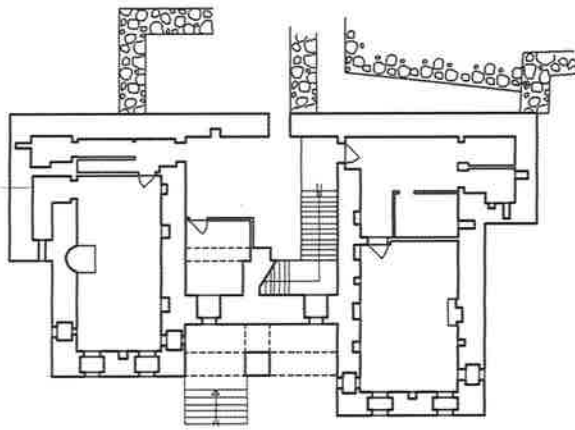
Resim 285. Ergeri'den kule tipi ev. Kat planları.
