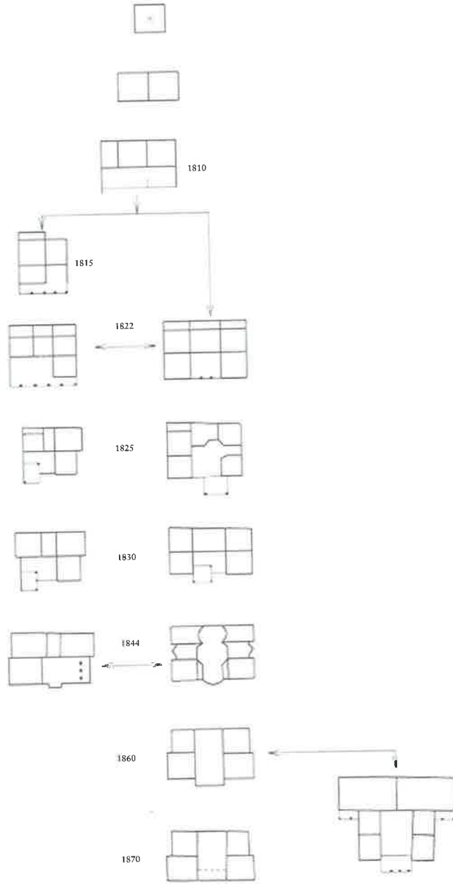
Resim 38. Bulgaristan geleneksel konut mimarisinde iç ve orta sofalı plan tipinin gelişimi.
