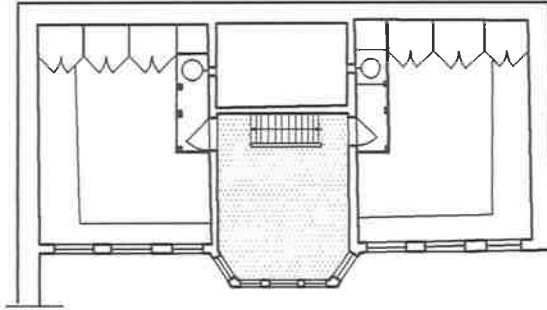
Resim 197. Bosna, Foča'dan bir evin kat planları.
