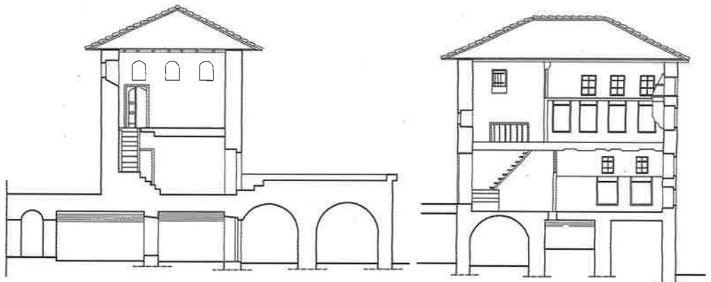
Resim 279. Berat'tan kule tipi ev. Kat planları, kesit ve görünüşler.
