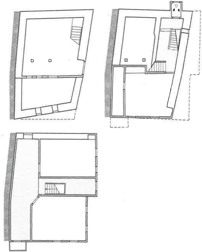
Resim 182. Ohri'de bir ev. Kat planları.
