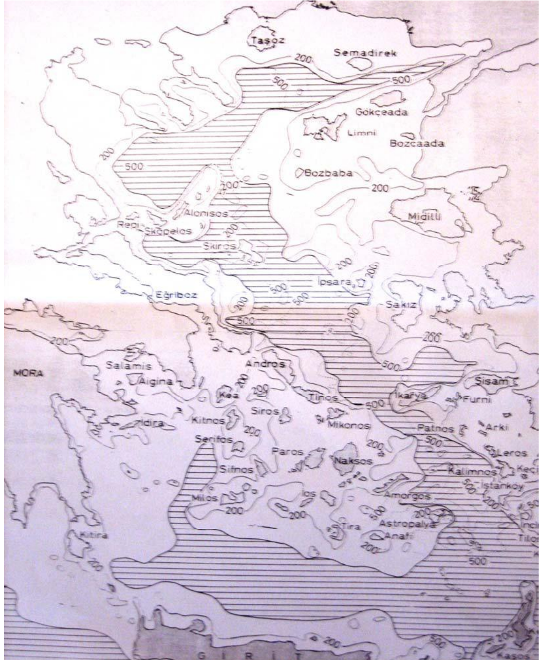
EK: I - Midilli Adası'nın Ege Adaları Arasındaki Konumu
