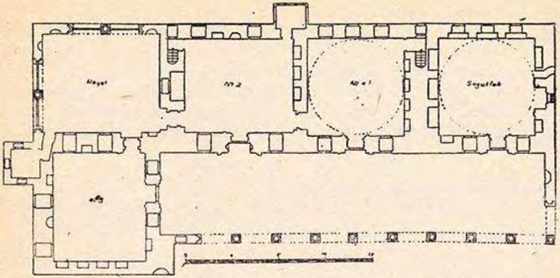
Fâtih Köşkü'nün plânı (Ekrem Hakkı Ayverdi arşivinden)
