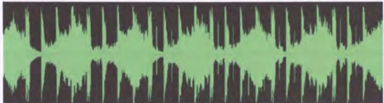
Ses dalgaları
