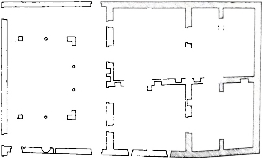
Resim 75: Karakabaklı'daki (Silifke) ev, plan.
