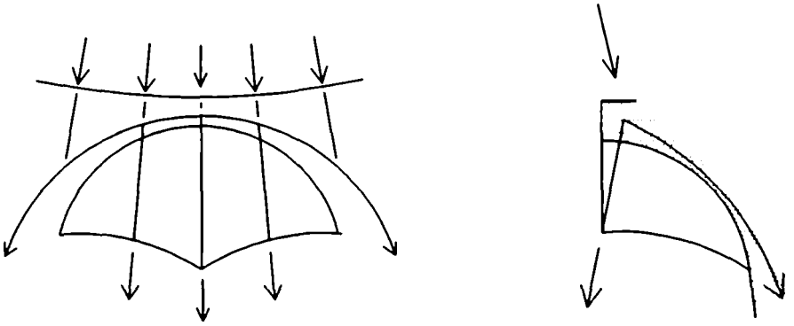
Resim 15: Trempita yörük tasarımı çizimi.
