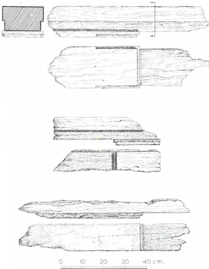
Resim 5: C Tipi kiriş.
