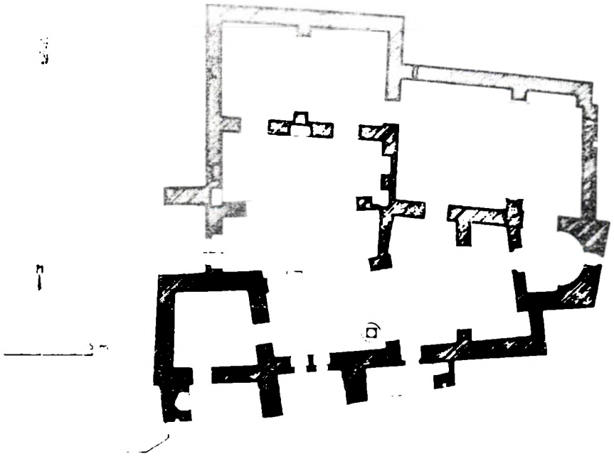
Resim 74: Sinekkaie'deki (Silifke) Bizans kervansarayı, plan.
