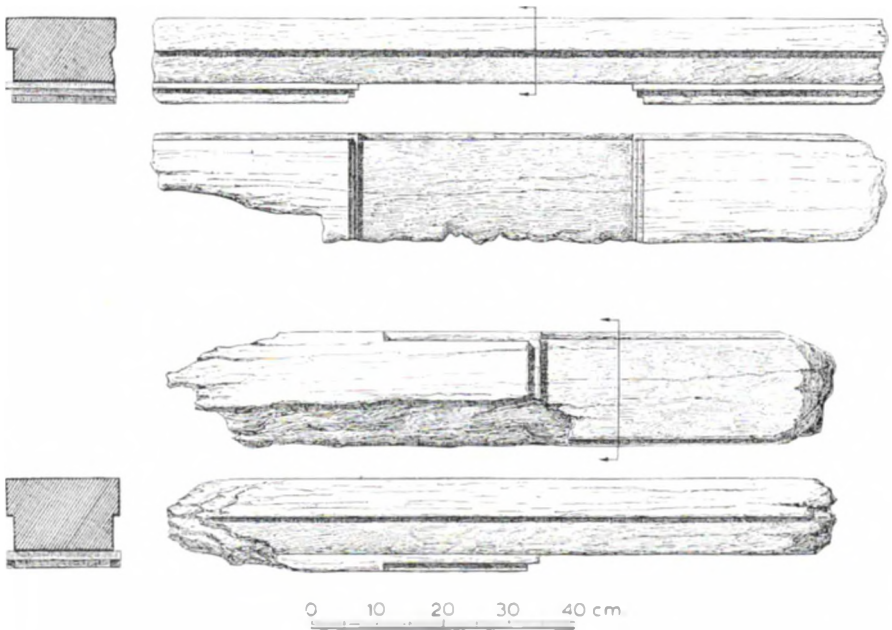
Resim 6: C Tipi kiriş.
