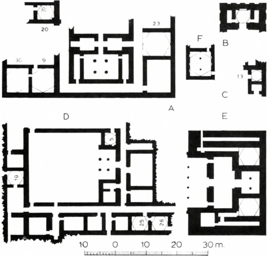
Resim 11: Orta Asya antik mimarlığında kırıışlı altıgen tonoz örnekleri.
