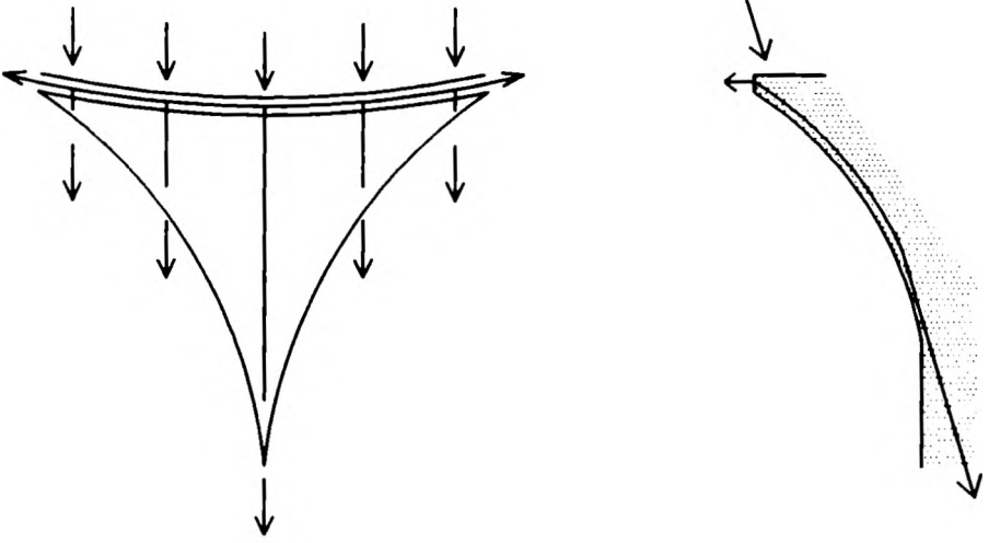
Resim 19: Pandantifte yük aklarını, çizim
