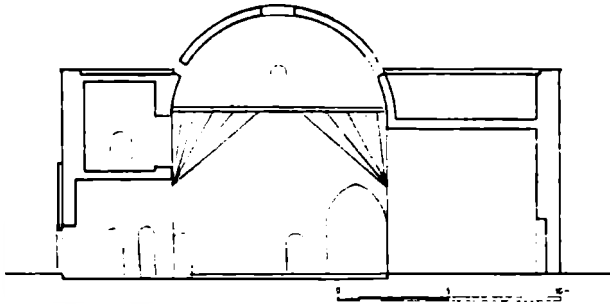
Resim 25: Karaman Ibrahim Bey Imareti, kat planları ve kesit. (M. Sozen, Anadolu Medreseleri II)
