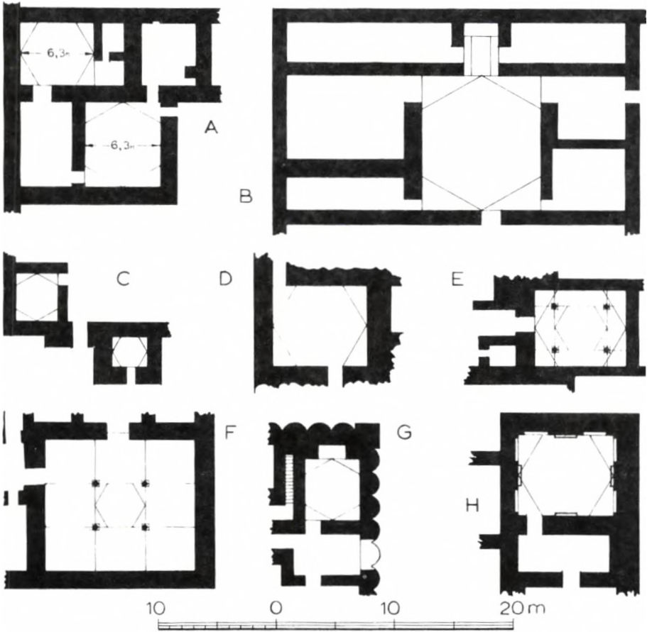
Resim 12: Erken Ortaçağ (Arap Öncesi) Orta Asya mimarlığında kirişli altıgen tonoz örnekleri
