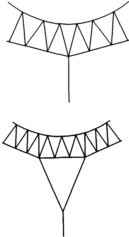
Resim 16: Üçgenler Kusagi çizimi.
