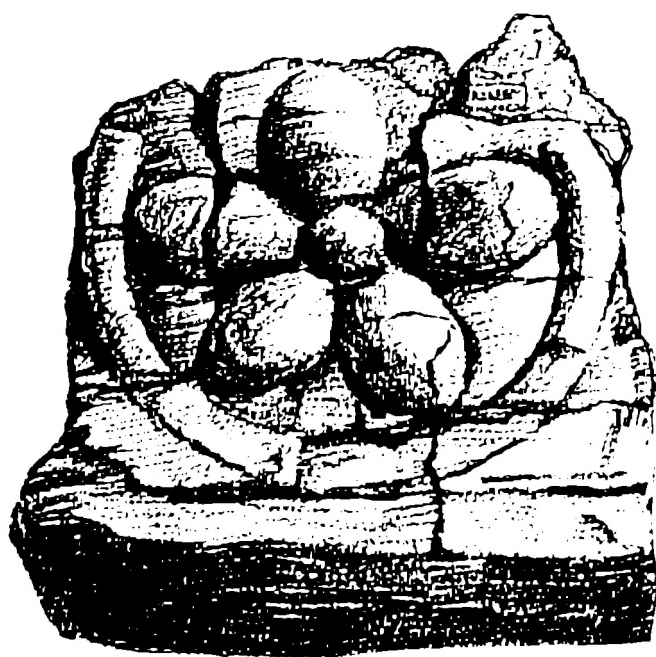
Resim 4a: B Trilete spores detay
