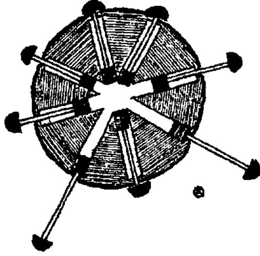
DEVİRİ DAİM BORUSUNUN ENİNE KESİTİ Ağırlıklar merkezkaç kuvvetiyle fırlayıp tam ortada bir vakum oluştururlar.
