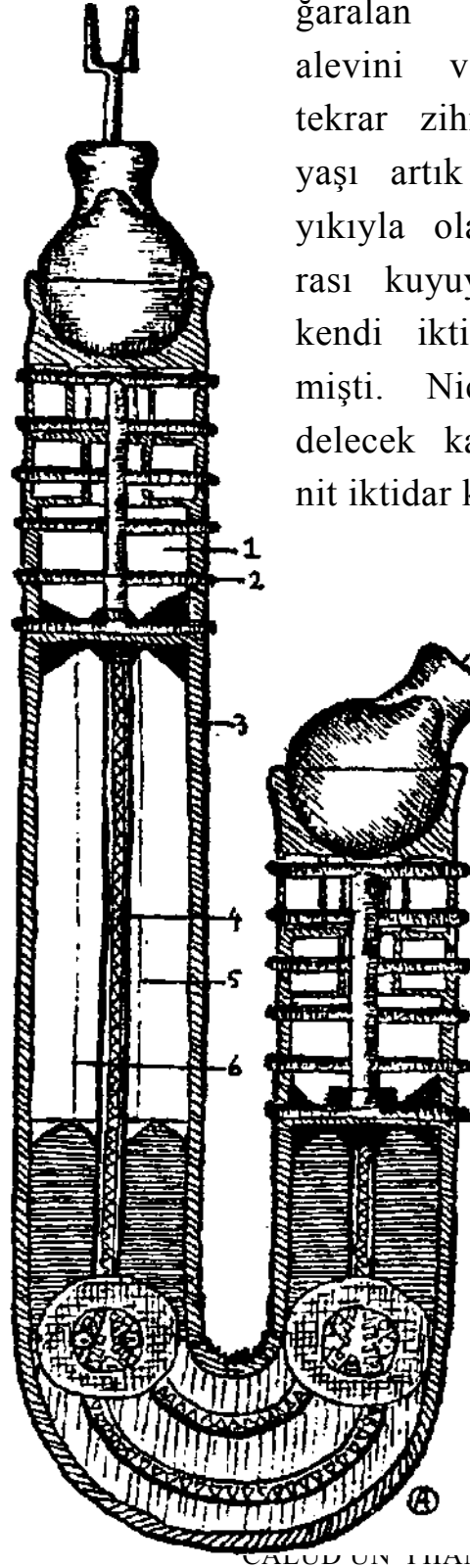
1- Makina dairesi. 2- Pençeler. 3-Gömlek. 4- âlimin, hiçbir güç kay- Omurga. 5- Kumanda telleri. 6- Pistona bu- harın basılmasını ve pistondan boşaltılmasını çağının sonsuz Ölmadl- sağıyan tel.
