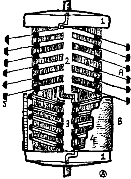
DEVİRİ DAİM BORUSU 1- Cıva dolu hazneler. 2-3- Cıvayı emen boşluklar, 4* Kılıf (boruyu bilezik gibi sarar ve boru tepetaklak olunca aşağıda kalır). 5- Pistonları çeken ağırlıklar. Boru eksenini etrafında dönmeye başlayınca ağırlıklar merkezkaç kuvvetiyle fırlayıp pistonları çeker. Oluşan vakum, cıvayı yukarıya çekince boru tepetaklak olur.
