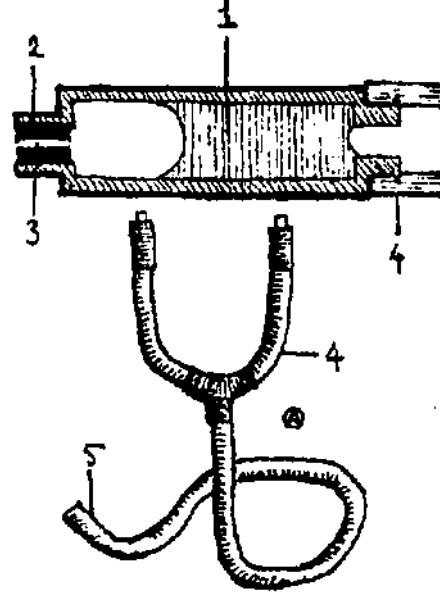
ÇİFT NAMLULU TOPLARI ATEŞLEME AYGITI
