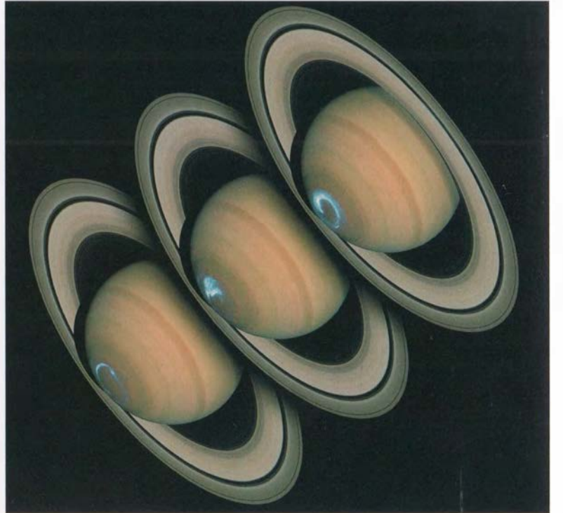
Aşağıda: Cassini uzay aracının, Hubble uzay teleskopuyla işbirliği sonucu gözlemlenen Satürn'ün halkaları ve kutup ışıkları.
