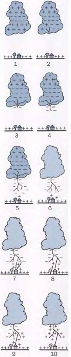
Yukarıda: Şimşek. (Açıklama için metne bakınız.)
