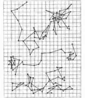
Yukarıda: Jean Perrin tarafından gözlemlenen Brown hareketi. Perrin sıvı çözelti içindeki üç adet sakızağacı reçinesi taneciğinin pozisyonlarını her 30 saniyede bir kaydetti ve zikzak hareketini gözler önüne sermek için pozisyonları düz çizgilerle birleştirdi. Bu deney atom ve moleküllerin varlığına ilişkin ilk inandırıcı delildi.
