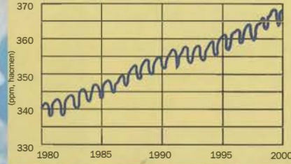
ATMOSFERDEKİ KARBONDİOKSİT
