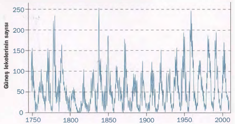
2001 başı
