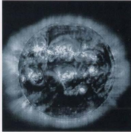
2001 başı
