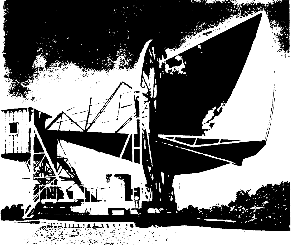
Şekil 1.8 : Şimdiye kadar yapılmış en duyarlı antenin şekli. Solda bağlandığı kulübede -235^{\circ}\text{C} 'ye kadar soğutulmuş bir yakut kristali vardır. Bu kristal kuvvetlendirici olarak ödev görmektedir 1960-1966 yıllarında atılan uyduların sinyallerini almak için geliştirilen bu alet, 13 milyar yıl önce Big-Bang ile ortaya çıkan radyo dalgalarını saptamaya başlamıştır.
