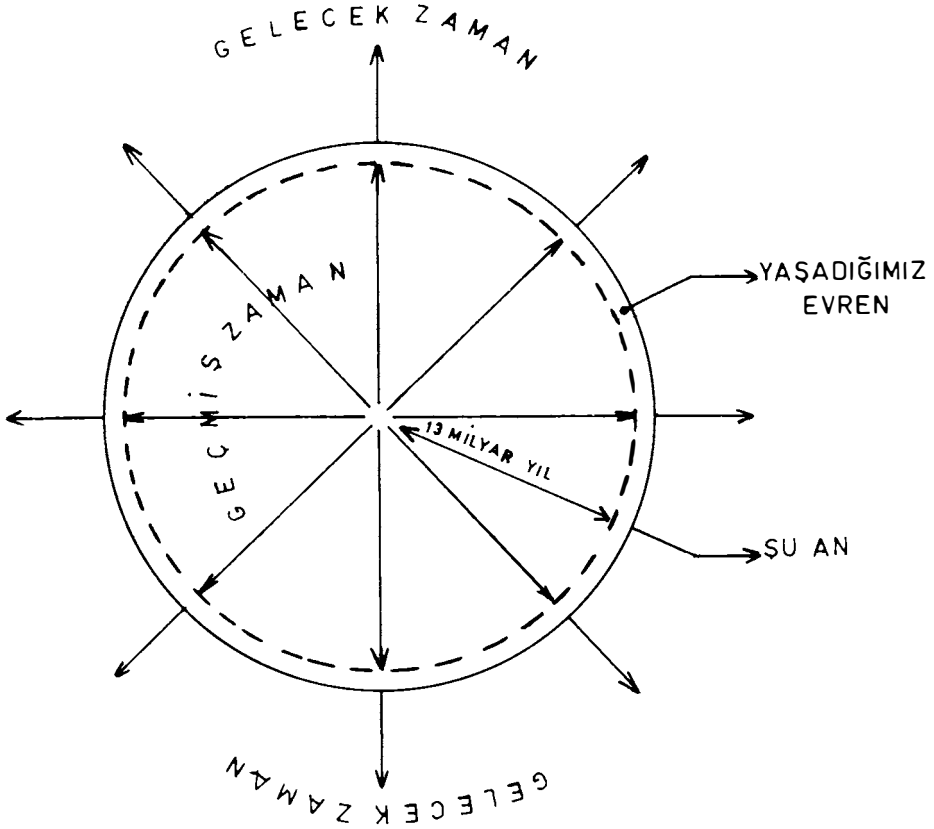
Şekil 1.7 : Uzak-zaman boyutu içerisinde evrenin kuramsal durumu.
