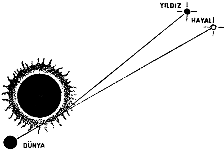
Şekil 1.4 : Yıldızdan gelen ışığın güneşin gravitasyon (kütleçekimi) alanında sapması. Güneşin gravitasyon (kütleçekimi) alanından geçerken yıldızın ışığı güneşe doğru saptığından, yıldızın görüntüsü dünya üzerindeki gözlemcilere göre güneşten dışarı doğru kaymış görünecektir.
