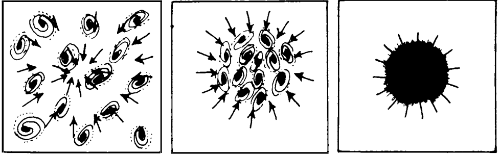
Şekil 1.10: Kapalı (sınırlı) evren modeline göre, genişleme durduktan sonra galaksiler birbirine doğru gitmeye başlar. Sol panel, galaksilerin birbirine doğru hareket etmesini gösteren oklarla dolu bir daireyi gösterir. Orta panel, galaksilerin birbirine doğru hareket etmesini gösteren oklarla dolu bir daireyi gösterir. Sağ panel, galaksilerin birbirine doğru hareket etmesini gösteren oklarla dolu bir daireyi gösterir.
