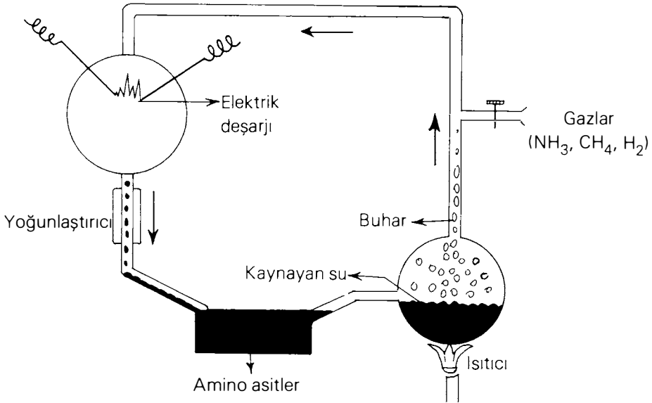
Şekil 2.1 : STANLEY MILLER'in dünyanın ilk evrelerindeki koşulları sağlayan aygıtı. Isıtılan suyun çıkardığı buharlar sağ taraftaki musluktan verilen gazlarla karışmakta ve sol taraftaki balonda bu karışım elektrik şarjı uygulanmaktadır. Oluşan amino asitler ve diğer organik bileşikler aşağıdaki hazinede birikmektedir.
