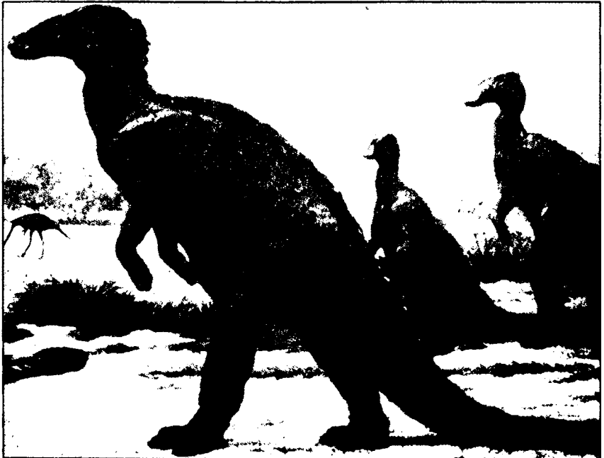
Şekil 14.25 : Kretase'den bir görünüm (Barnes'den).
