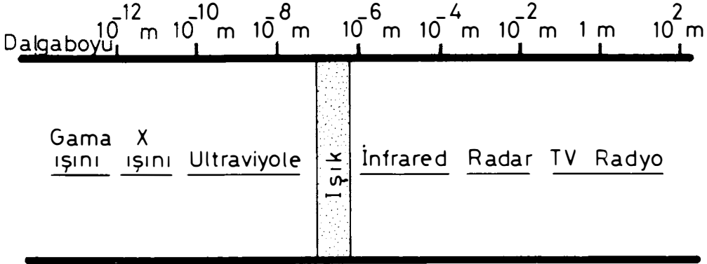
Şekil 1.16: Elektromanyetik spektrum.
