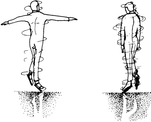
Şekil 1.12: Kendi etrafında dönen buz patencisi, kollarını vücuduna doğru çektiğinde, hızı artar; bu şekilde açısal momentumu korunmuş olur.
