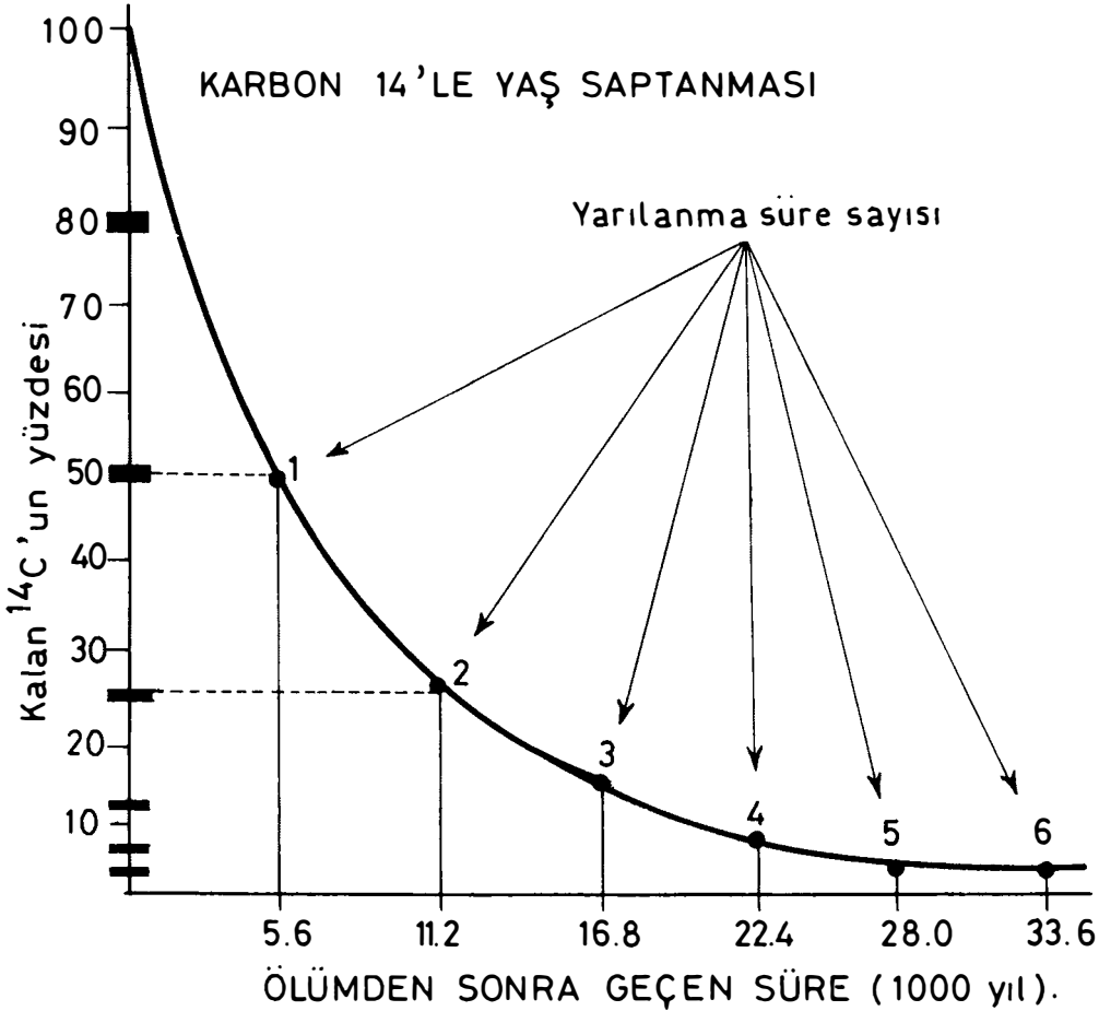
Şekil 14.1: Karbon-14'ün yarılanma süresi yaklaşık 5.600 yıldır. Bir canlı öldüğünde, içerdiği karbon-14'ü bu hızla yitirir. Eğer bir fosil, orijinal karbon aktivitesinin % 20'sini gösteriyorsa, bu fosilin yaşı 13.250 yıldır.
