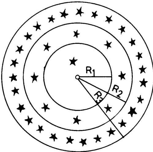
Şekil 1.5: OLBERS paradoksu. R, her 10 ışık yılını göstermektedir.
