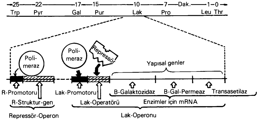
Şekil 11.73: Lak-operonunun ve regülatör geninin şeması. Üstte koli haritasının büyük bir kısmı (Bresch ve Hausmann'dan).
