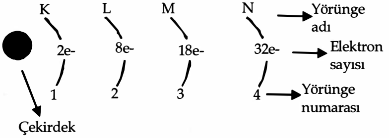
Elektronların yörüngelere göre konumlanması
