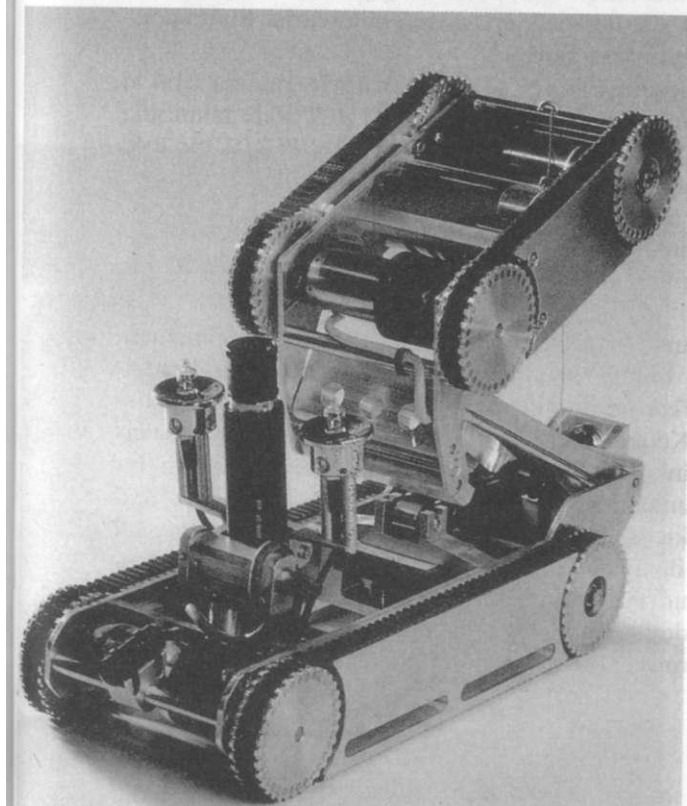
Rudolf Gantenbrink tarafından imal edilen robot "UPUAUT".
