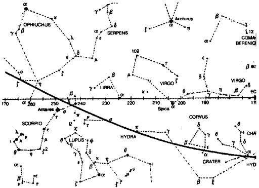
5.4. Bahar ekinoksu Boğa takımyıldızındayken gökyüzü ekvatoru (yalnuzca antik dönemde bilinen takımyıldızlar gösterilmiştir)
