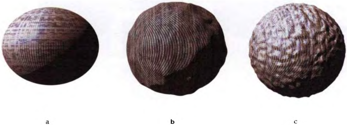
Şekil 3.17 Olası ve Olanaksız Geçmişler
