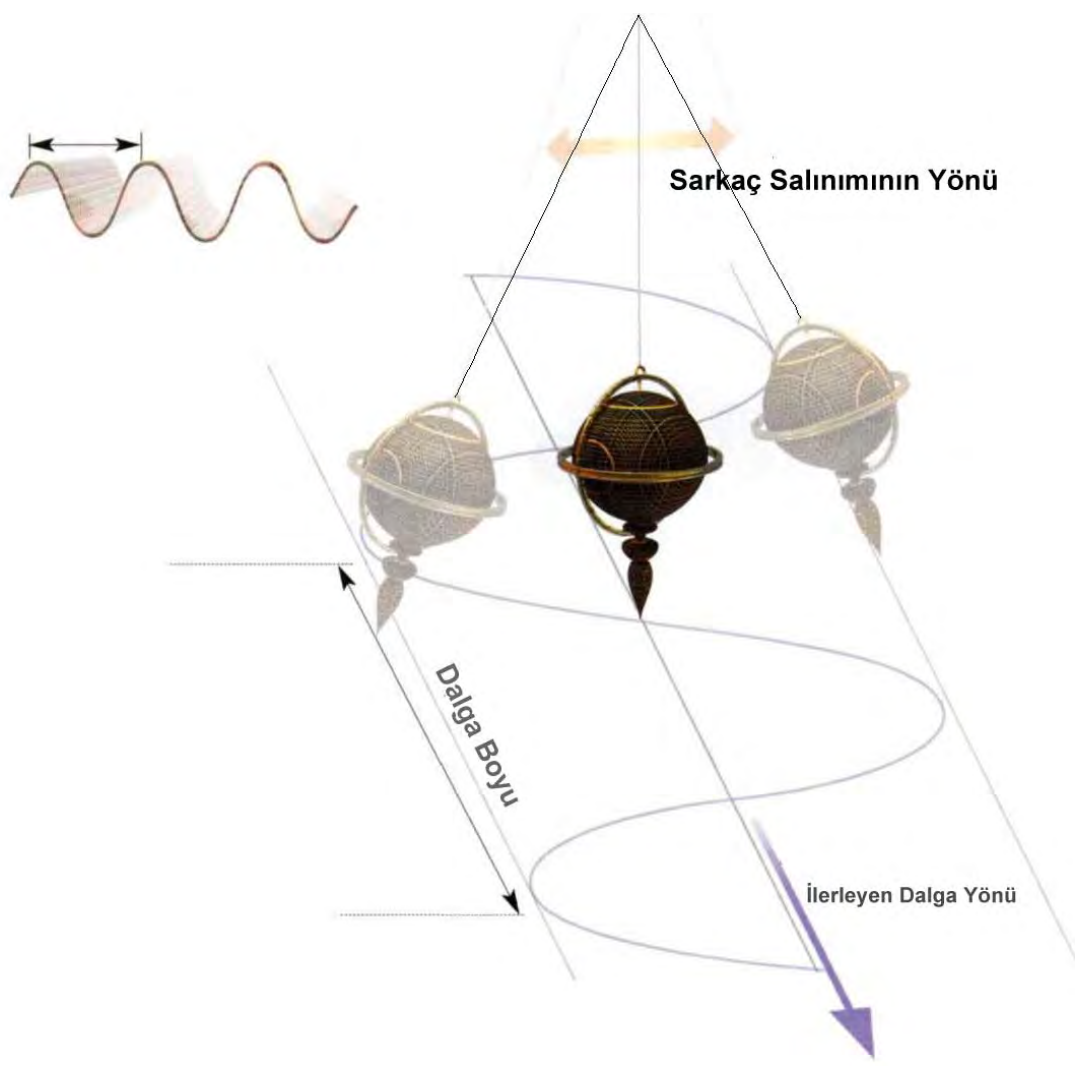
Şekil 2.9 İlerleyen İle Salınan Sarkacın İlişkisi
