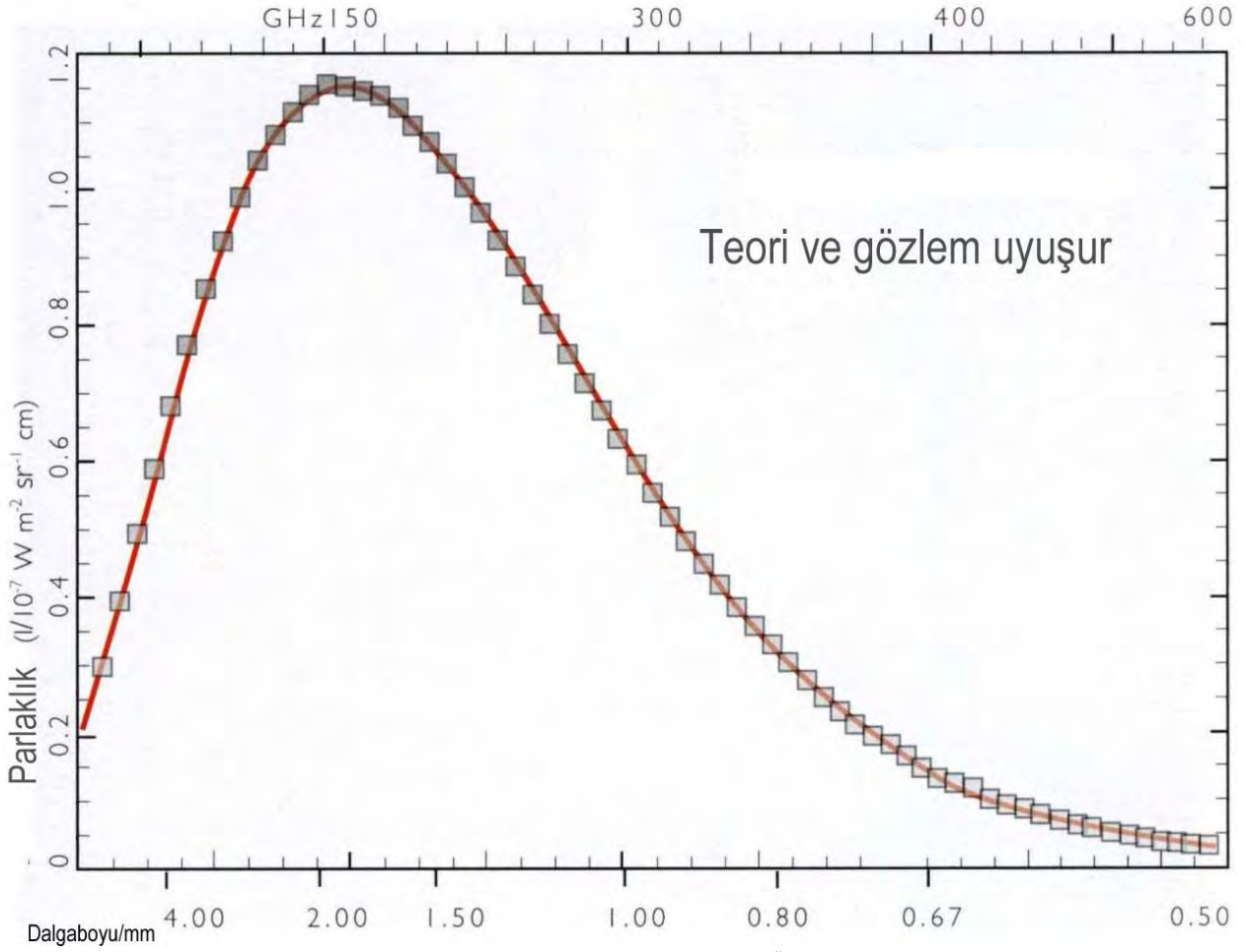
Şekil 2.6 Mikrodalga Fon Tayfının Ölçümü
