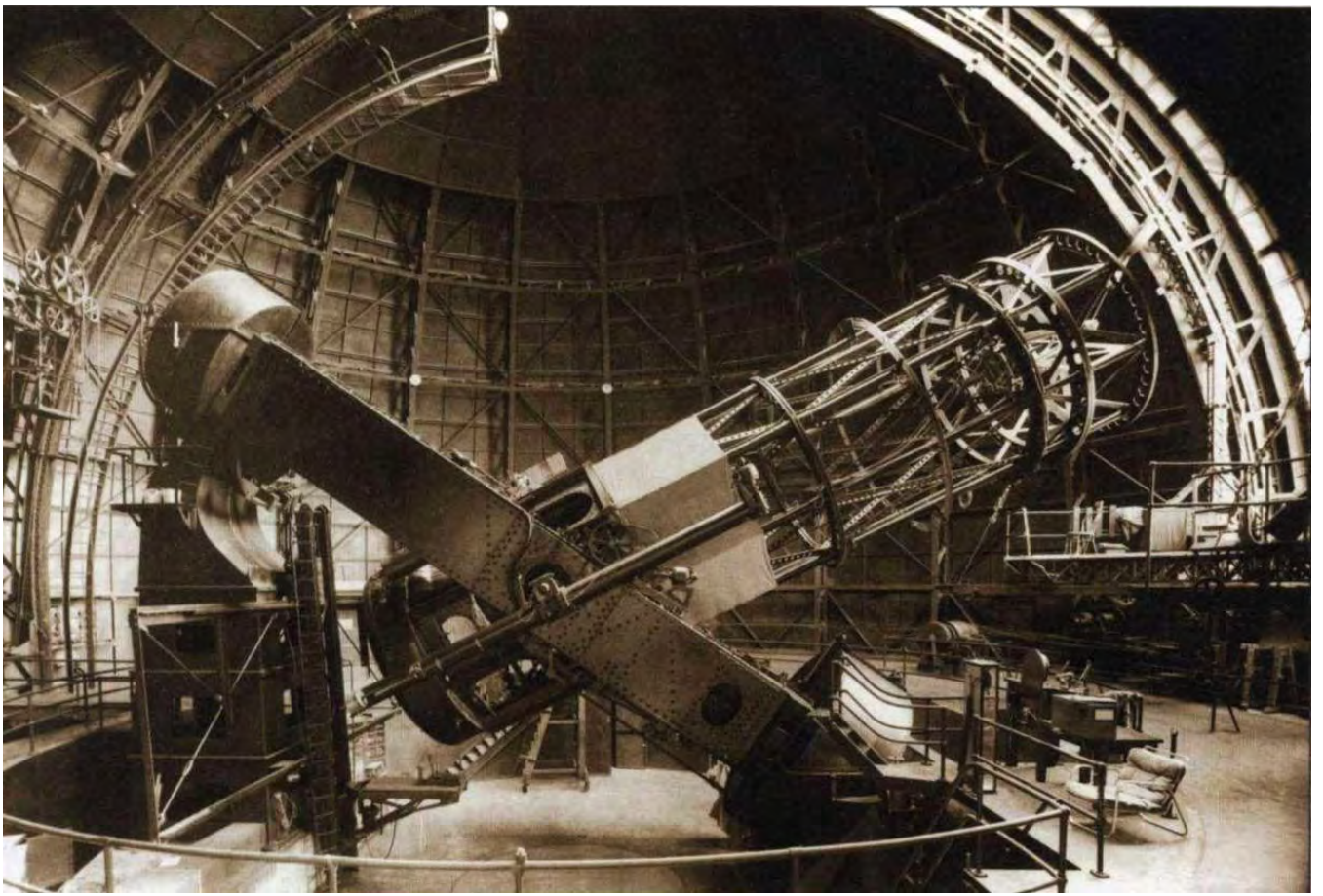
Mount Wilson Gözlemevi'ndeki 100 Hooker teleskopu.
