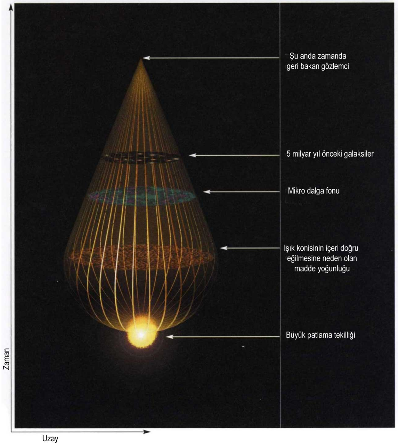
Şekil 2.8 Zaman Armut Biçimindedir
