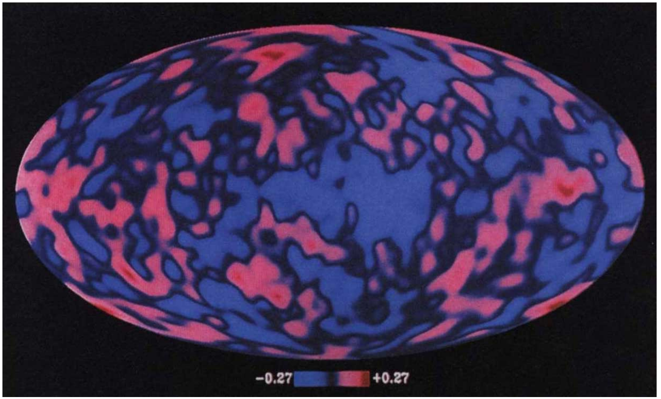
COBE uydusu DMR aracı ile yapılan gökyüzünün tam haritası zamandaki kırıxıklıklar için bir kanıt sunuyor.
