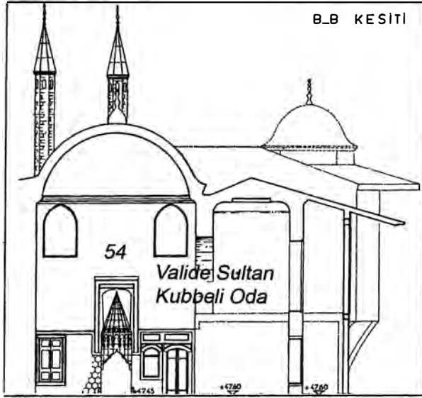
Levha 8. Harem, Valide Sultan'a ait mekânlar, kesit Eldem-Akozan, (Lev. 6/54)
