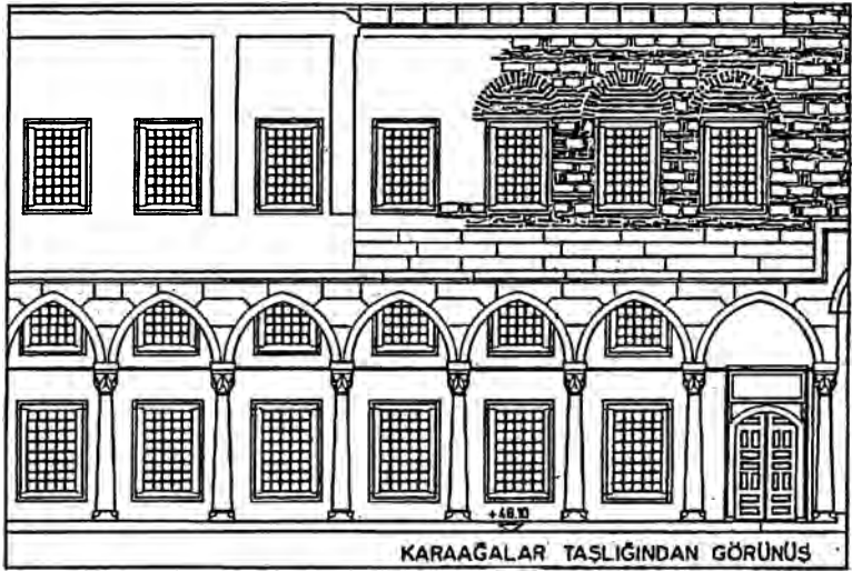
Levha 14. Kara Ağalar Koğuşu, kesit; Eldem-Akozan 1982
