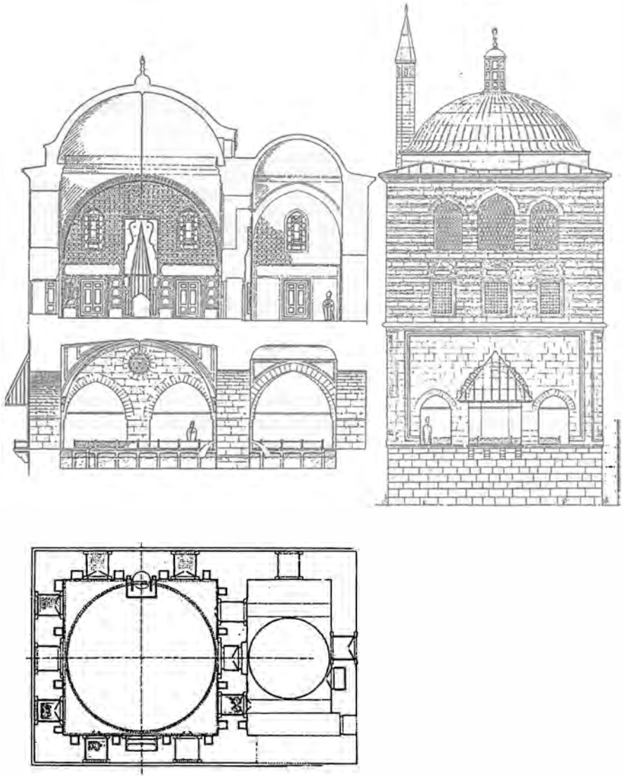
Levha 18. III. Murad Odası, plan ve kesit; Eldem-Akozan 1982
