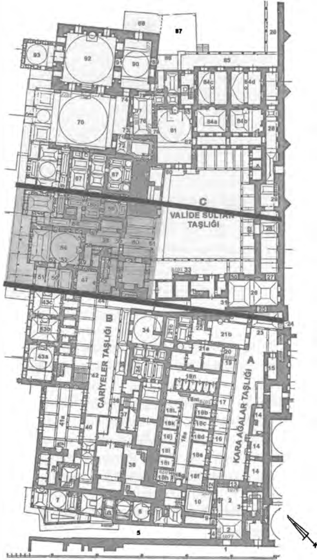
Levha 9. Valide Sultan'a ait mekânların harem içindeki konumu, plan, Eldem-Akozan, 1982.
