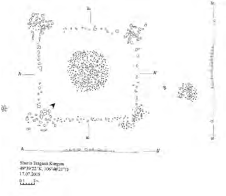
Foto XX. Sarıngöl EDÇ Kırigsuru Çizimi
